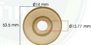
■ HG381-81 Clutch Cover ฝารองคลัทช์
