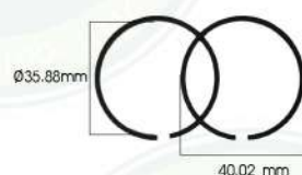
■ HG180-70 Pipe ring แหวนท่อนลม
