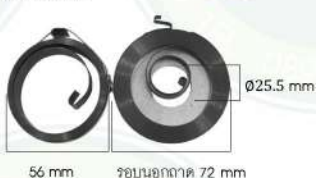
■ HG52-115 Starter spring EZ สปริงสตาร์ท EZ
